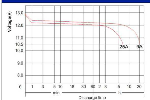
Curva di scarica T-A ( 25°C,70°F )
